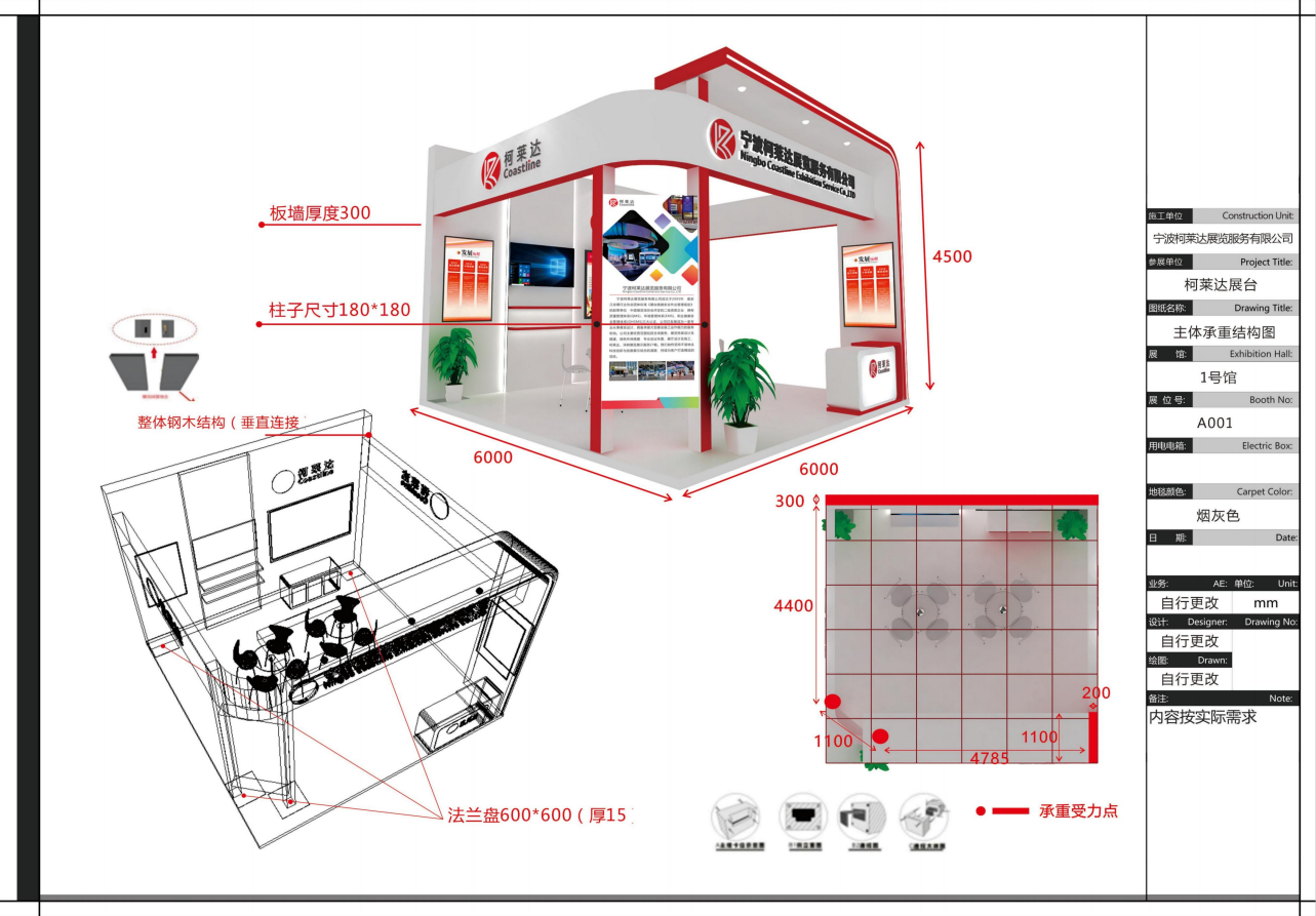
主体结构承重图
